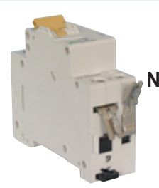
Одинаковый соединительный угольник ZV-N-05TE (-80A) для N(PL6 с 1,5MU) 50 и 80A шиной
