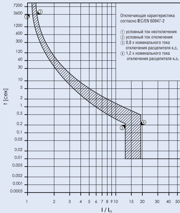
Кривая отключения VZM1 32А, 3-х полюсное исполнение
