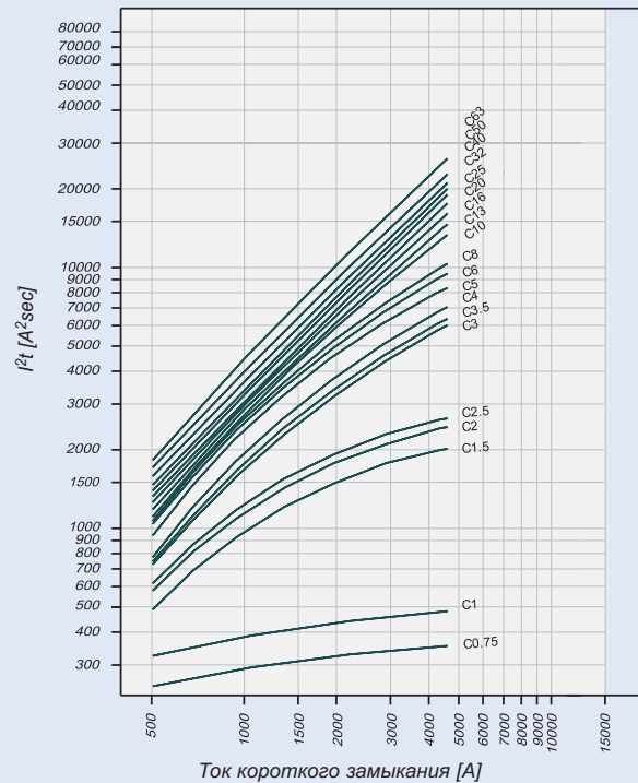
Характеристика I 2 t, характеристика отключения C, 1-полюсное исполнение
