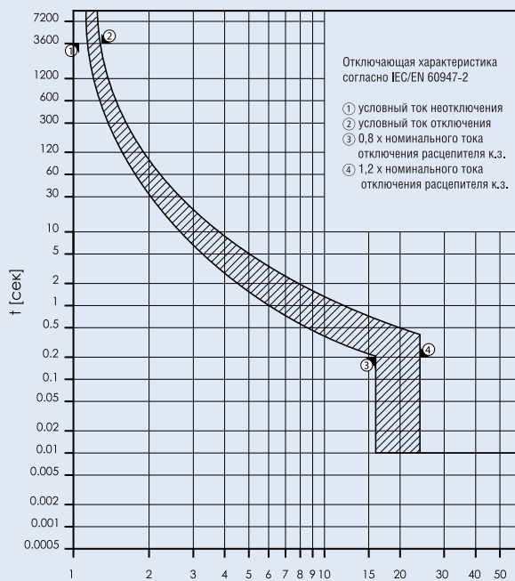
Кривая отключения VZM1 16А, 3-х полюсное исполнение
