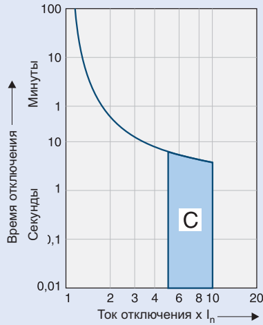
Характеристика отключения C (расцепитель короткого замыкания 5 – 10 I n )
