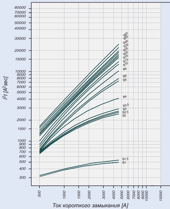
Характеристика I 2 t, характеристика отключения B, 1-полюсное исполнение
