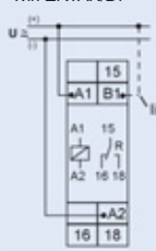
Тип ZRMF2/WBt
