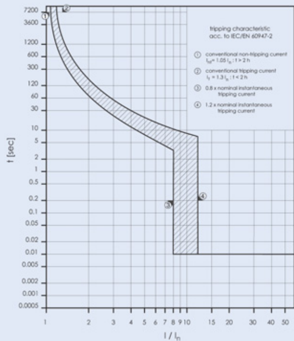
Кривая отключения VZM2 125A
