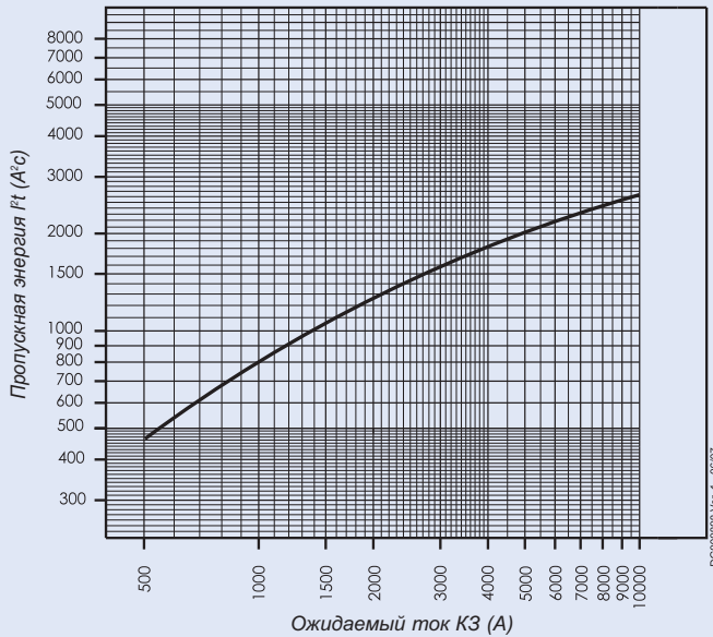
Тип FAZ...-HS
