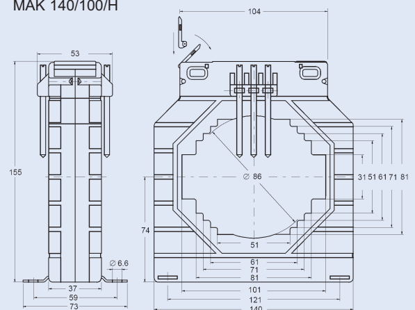
MAK 140/100/H
