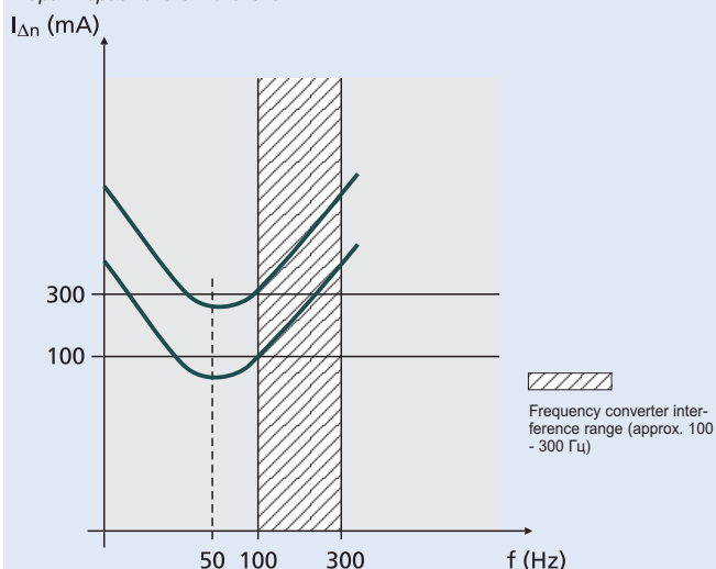
Характеристика отключения
